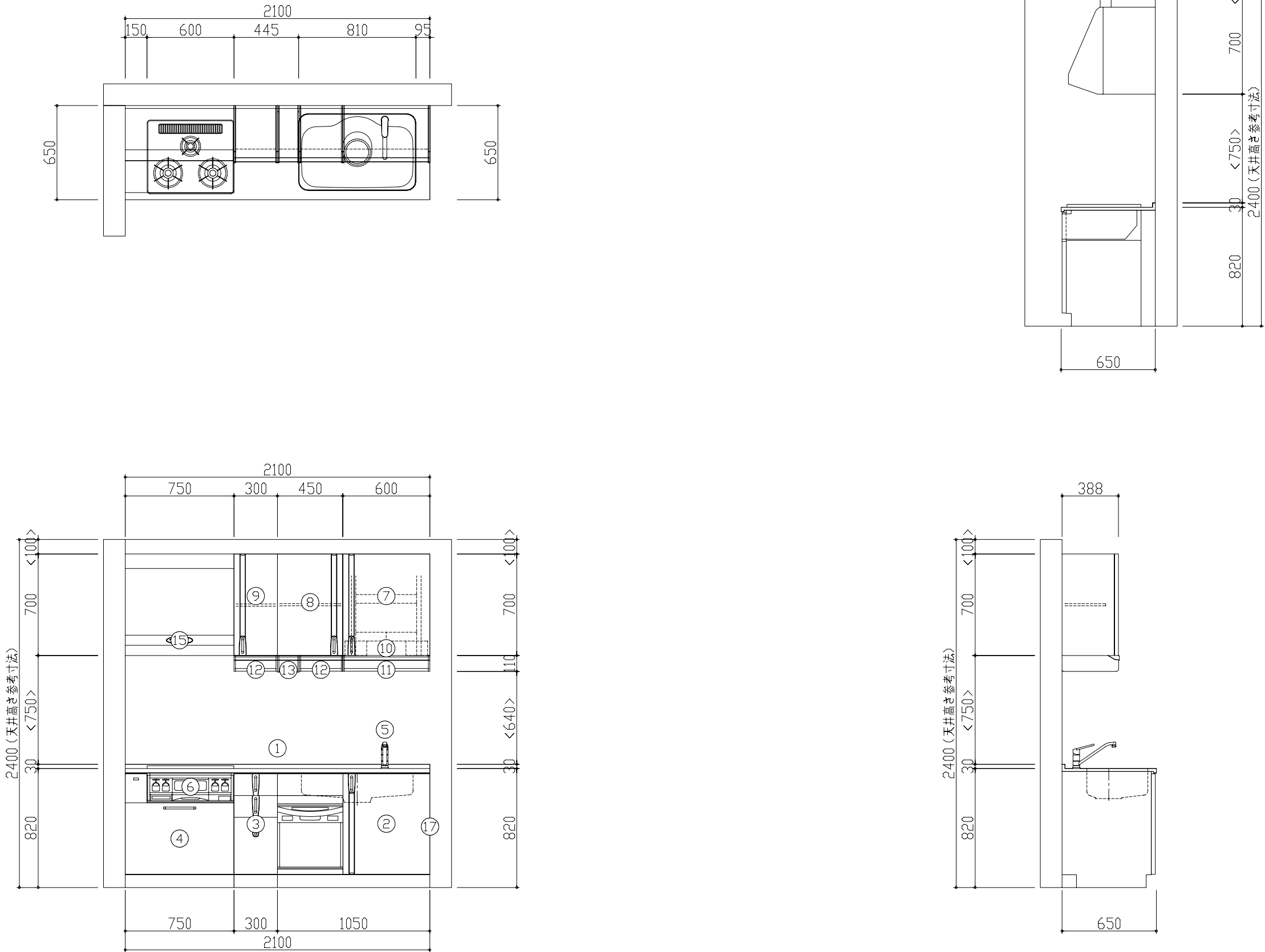
A正面図 B側面図
